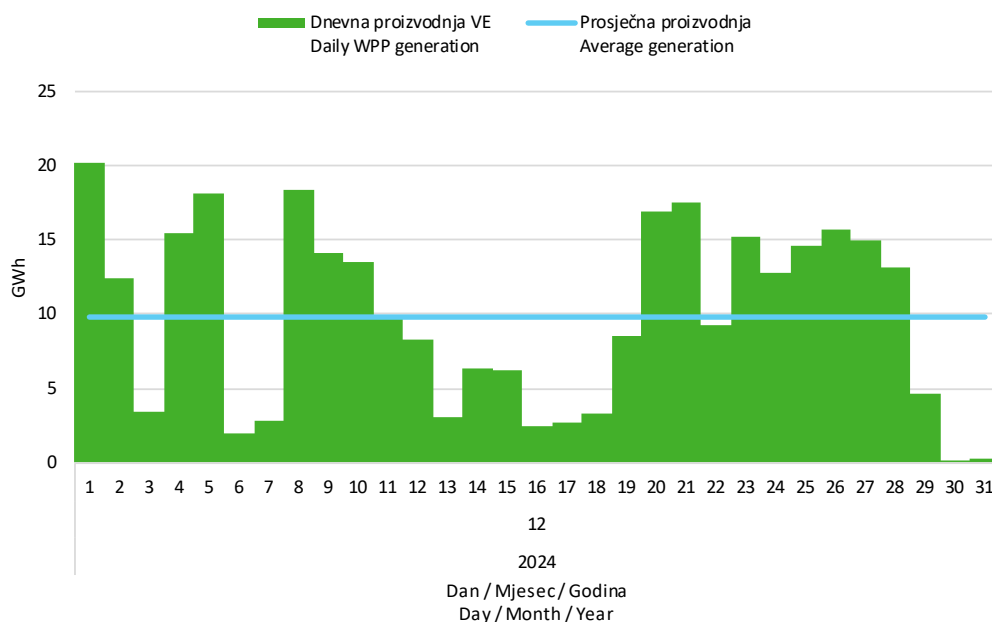
Slika 5 Dnevna proizvodnja svih vjetroelektrana u prosincu 2024. godine
