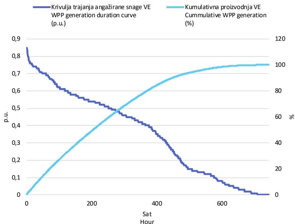
Slika 3 Krivulja trajanja angažirane snage svih VE i kumulativna proizvodnja VE u prosincu 2024. godine u jediničnim vrijednostima
