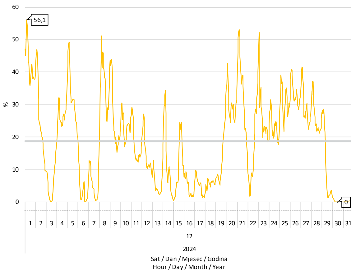
Slika 8 Udio proizvodnje vjetroelektrana u pokrivanju satnog opterećenja elektroenergetskog sustava u prosincu 2024. godine
