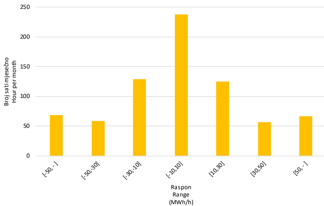
Slika 10 Statistička raspodjela satnih promjena proizvodnje VE u prosincu 2024. godine
