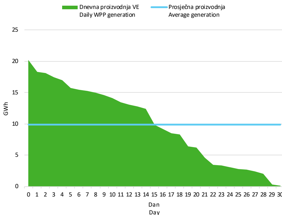
Slika 6 Krivulja trajanja dnevne proizvodnje vjetroelektrana u prosincu 2024. godine
