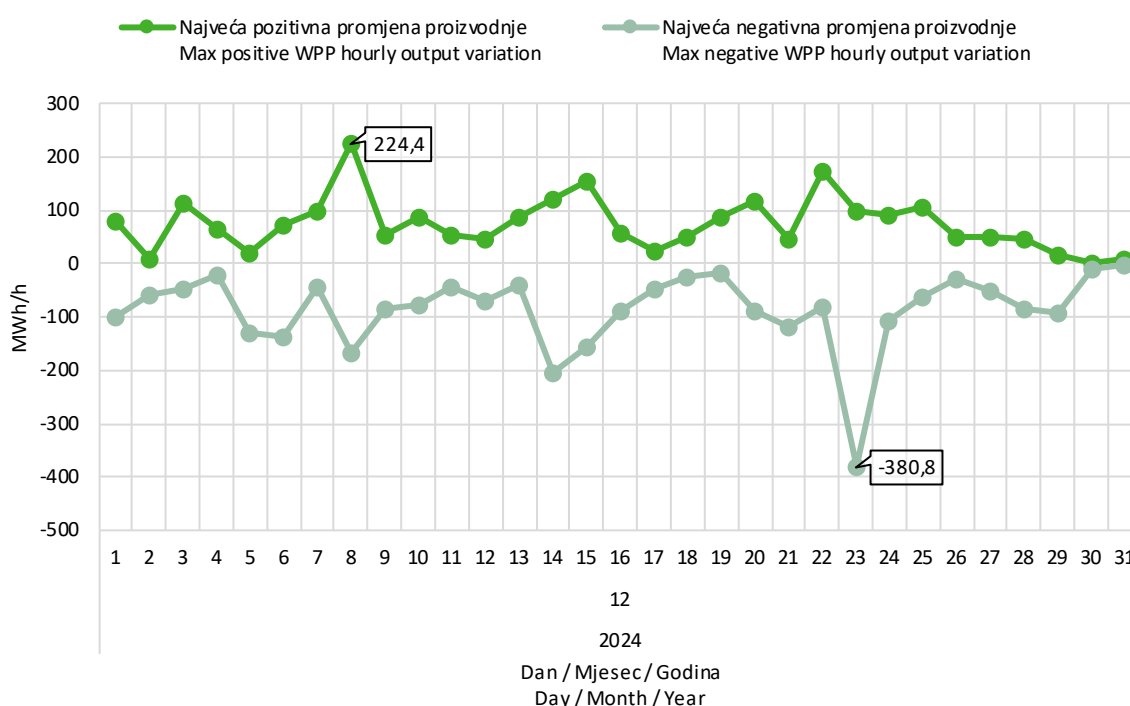
Slika 9 Maksimalna pozitivna i maksimalna negativna promjena satne proizvodnje VE u prosincu 2024. godine
