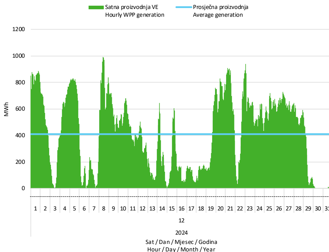
Slika 2 Satna proizvodnja svih vjetroelektrana u prosincu 2024. godine
