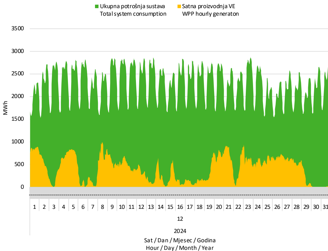
Slika 7 Usporedba satnog dijagrama opterećenja sustava i proizvodnje vjetroelektrana u prosincu 2024. godine
